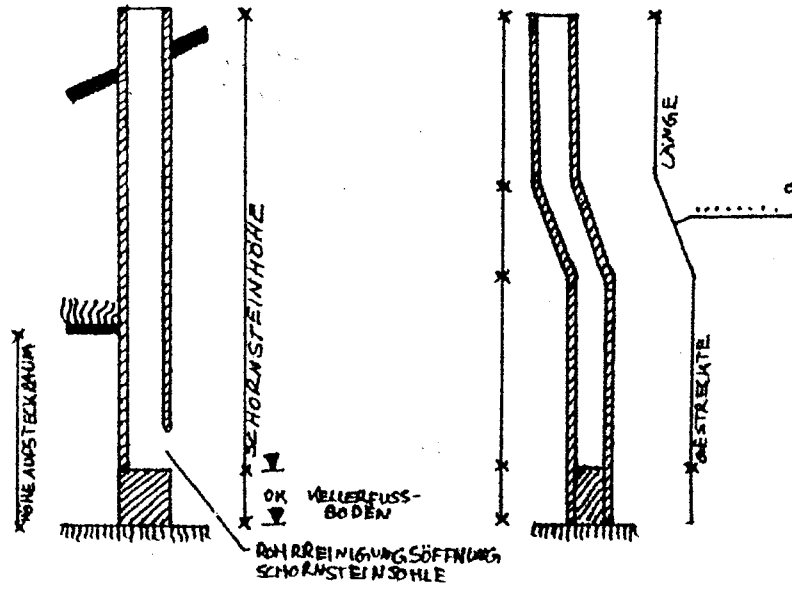
HEIZRAUMSKIZZE MIT KESSELSTANDORT UND LAGE DER T-STÜCKE, REINIGUNGEN, KONDENSATABLÄUFE
